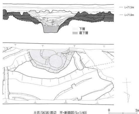
図3:SK38 平面図・断面図
